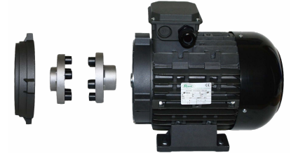
空心轴+内置弹性联轴器 三相 - 四级 (1450 RPM)
